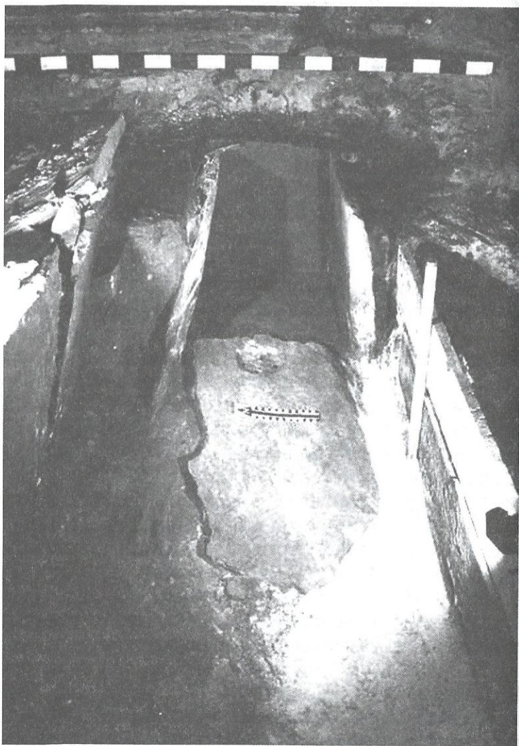
Рис. 42. Шиферний саркофаг з отвором для стоку рідини (Успенський собор Києво-Печерського монастиря).
